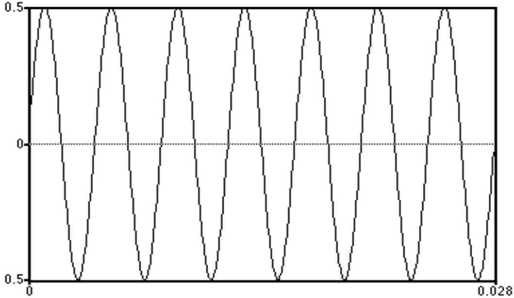
شكل 1. 3 - موجة صوتية ذات تردد مرتفع
